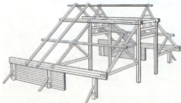
Рис. 12. Конструкция гумна в Красной Звезде Клецкого р-на
