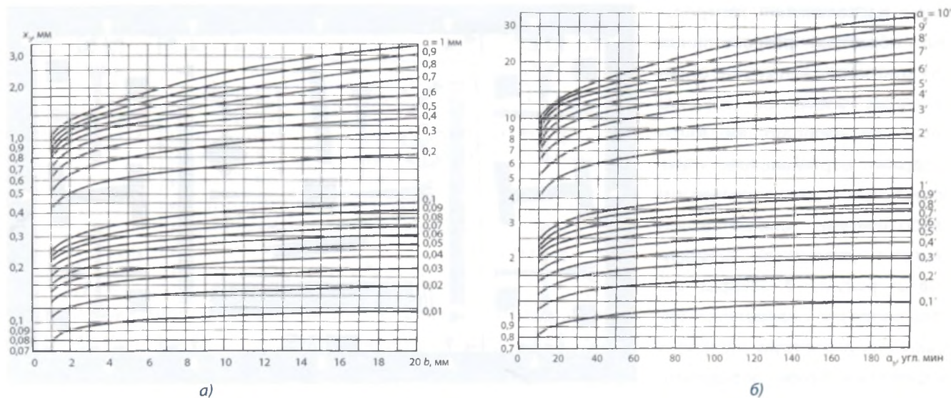
Рисунок 3 – Номограммы для определения эквивалентного размера протяженных объектов различения при расстояниях от глаза до объекта: а) – до 500 мм; б) – более 500 мм
