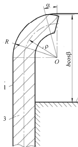
Рис. 3. Схема копирования заготовкой контура пуансона за счет локальной потери ее устойчивости
