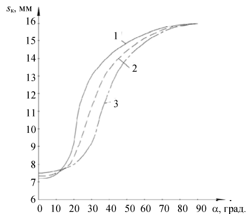
Рис. 5. Зависимости толщины \delta_k краевой части стенки заготовки при ее раздаче от угла контакта с пуансоном для разных коэффициентов контактного трения: 1 — f = 0,2 ; 2 — 0,3 ; 3 — 0,4
