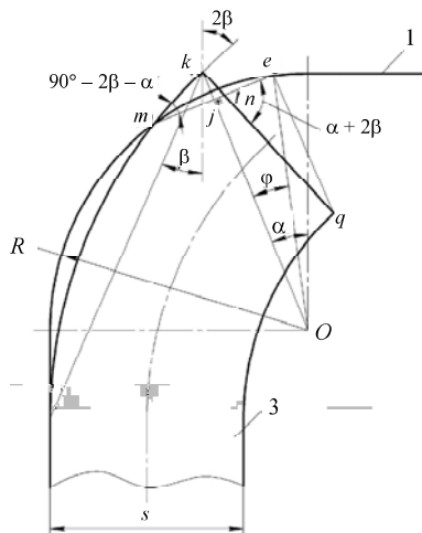
Рис. 4. Схема для определения геометрических параметров формоизменения кромки трубной заготовки при ее раздате
