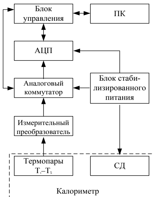
Рисунок 10 – Блок-схема установки для измерения тепловых характеристик СД
