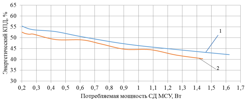
Рисунок 5 – Зависимости энергетического КПД от потребляемой мощности
