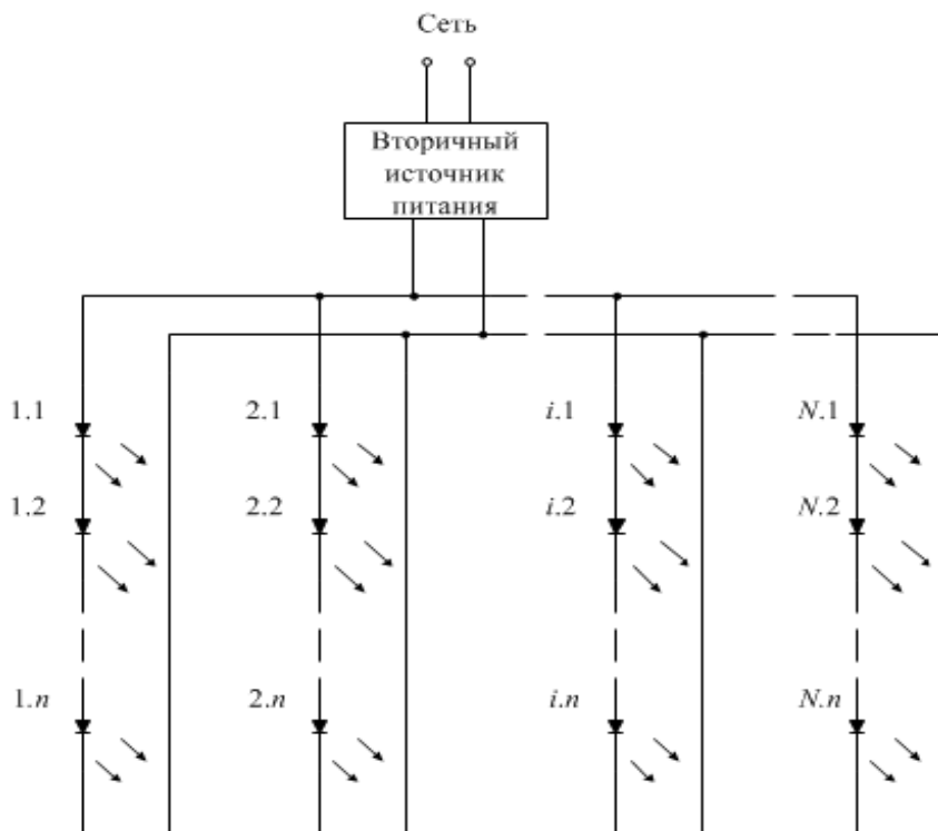
Рисунок 4 – Схема MCU на основе СД ARPL-1W White 6000
