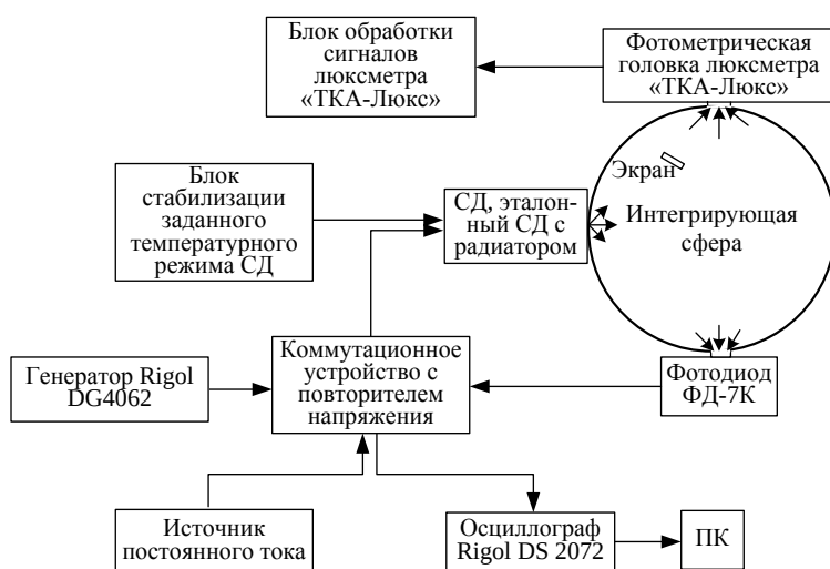
Рисунок 11 – Структурная схема испытательного фотометрического стенда
