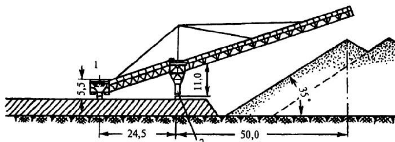
Рис. 5.5. Схема работы штабелеукладчика: 1 – ходовая тележка; 2 – приводная тележка
