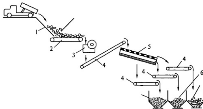
Рис 3.1б. Простейший дробильно-сортировочный завод: 1 — приемный бункер; 2 — питатель; 3 — дробилка; 4 — ленточные транспортеры; 5 — грохот; 6, 7, 8 — бункера для мелкого, среднего и крупного продуктов дробления
