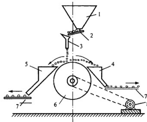
Рис 3.9б. Избирательное обогащение каменных материалов на механическом классификаторе (сепараторе): 1 — бункер; 2 — питатель; 3 — точка; 4 — воронка для материала пониженной прочности; 5 — то же, повышенной прочности; 6 — классифицирующий барабан; 7 — транспортеры; 8 — электродвигатель.
