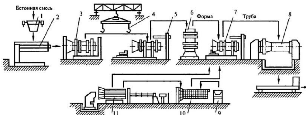
Рис. 6.31. Технологическая схема изготовления труб методом центрифугирования: 1 – раздаточный бункер; 2 – ленточный питатель; 3 – центрифуга; 4 – траверса; 5 – стенд; 6 – консольные съемники; 7 – форма на посту тепловой обработки; 8 – пост разборки, чистки, смазки; 9 – установка для испытания труб; 10 – станок для изготовления фиксаторов арматуры; 11 – стенд для сборки двойных арматурных каркасов.
