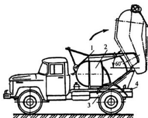
Рис. 6.17. Автобетоновоз: 1 — крышка; 2 — кузов; 3 — шарнир; 4 — рама.
