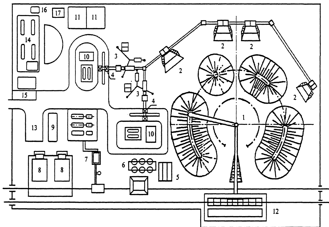
Рис. 3.1. Генеральный план прирельсового АБЗ
