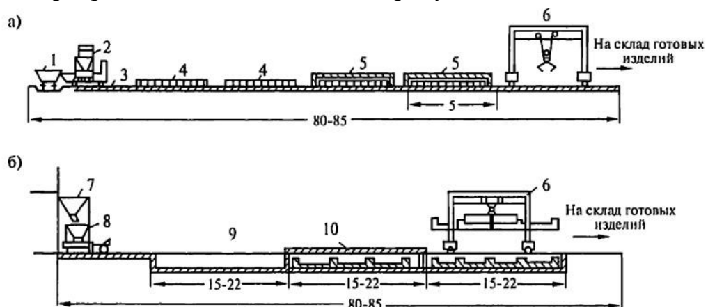
Рис. 6.23. Технологическая линия формования изделий с применением портального крана
