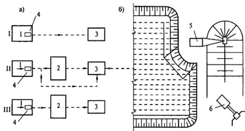
Рис 2.9. Схемы разработки карьера песчано-гравийных месторождений:
