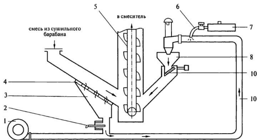
Рис. 5.14. Технологическая линия для получения трибоактивированных песков: 1 – вентилятор; 2 – шиберная задвижка; 3 – приемный бункер песка; 4 – вибрирующая металлическая сетка; 5 – горячий элеватор; 6 – устройство для подачи ПАВ; 7 – емкость для ПАВ; 8 – циклон; 9 – дроссельная заслонка; 10 – трубопровод-активатор.
