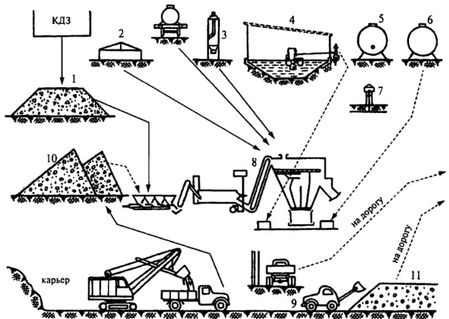
Рис. 5.18. Схема технологического процесса приготовления черного щебня:
