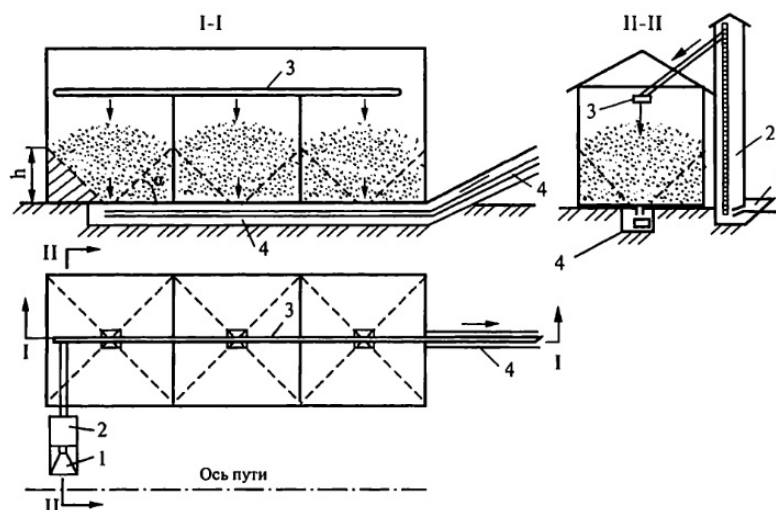
Рис. 5.7. Схема амбарного и бункерного (пунктирные линии) складов:
