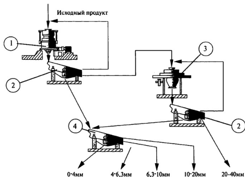
Рис 3.7а. Технологическая схема получения кубовидного щебня: 1 — конусная дробилка; 2 — двухситный грохот; 3 — центробежная дробилка; 4 — трехситный грохот.
