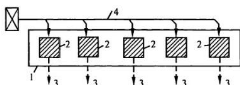
Рис. 6.21. Стендовая технологическая схема полигона: 1 – стенд; 2 – посты изделий (неподвижные); 3 – перемещение готовых изделий на склад; 4 – подвижное технологическое оборудование для армирования, формования и других операций.
