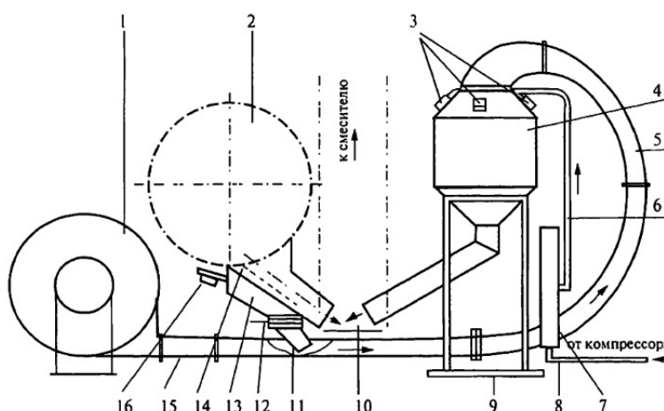
Рис. 5.15. Опытно-промышленная установка для трибоактивации песков:
