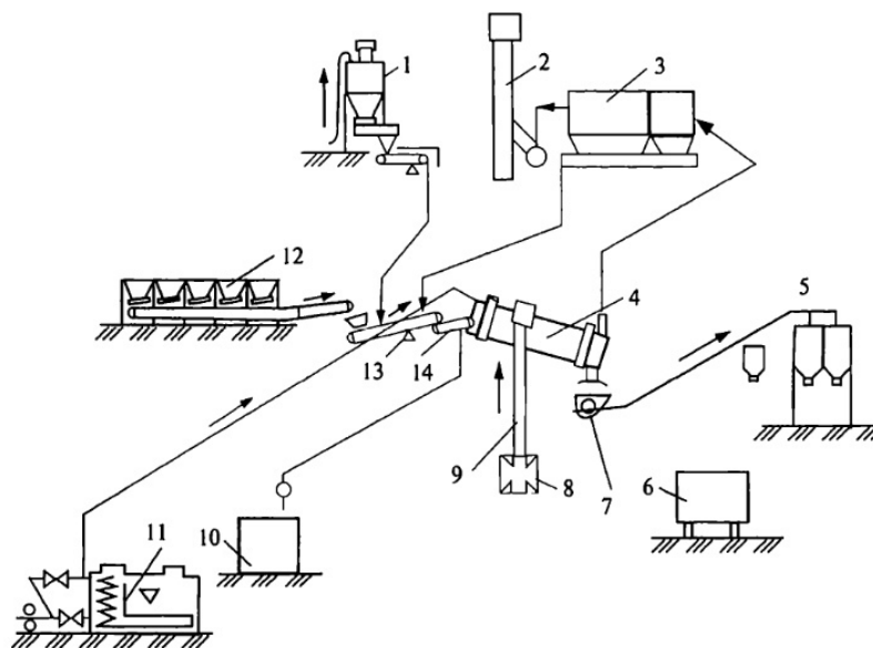
Рис. 5.20. Технологическая схема специальной асфальтосмесительной регенерационной установки:
