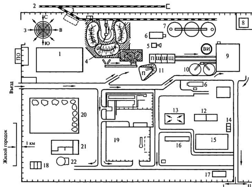
Рис. 6.3. Генеральный план ЦБЗ:
