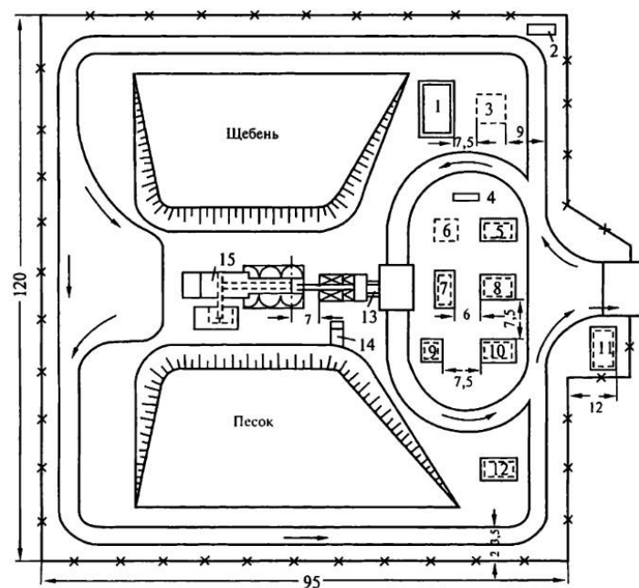
Рис. 6.2. Генплан притрассового бетонного завода:
