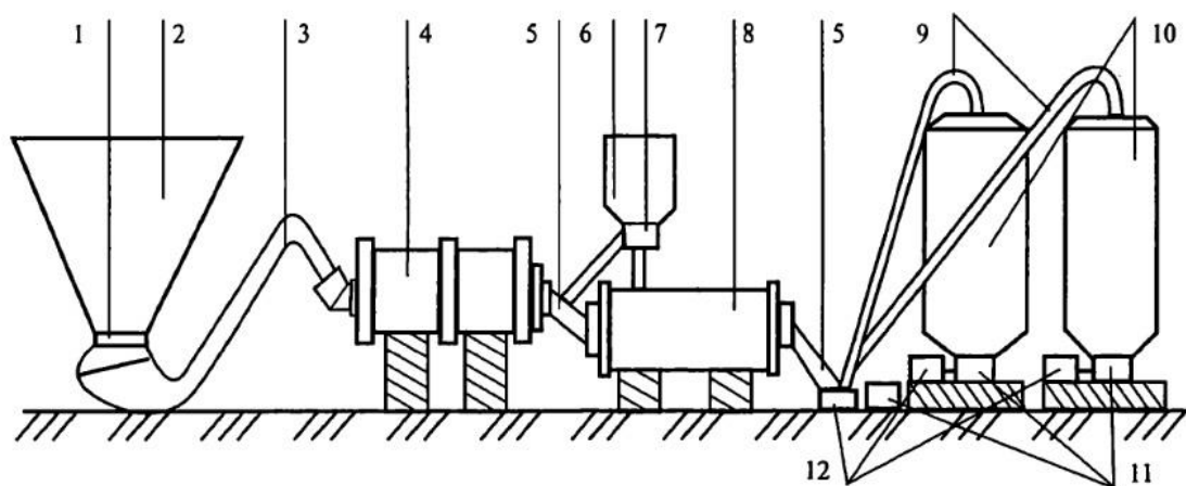
Рис. 5.13. Технологическая схема получения активированного минерального порошка из ОФС:
