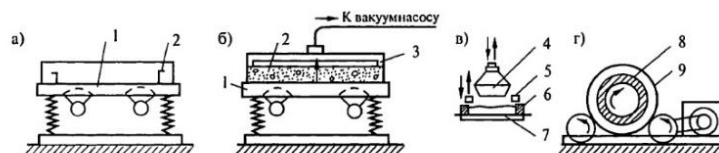
Рис. 6.30. Схемы уплотнения бетонной смеси в изделиях:
