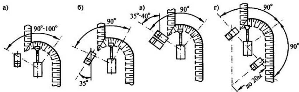
Рис 2.8. Схемы подачи автомобилей-самосвалов под погрузку:
