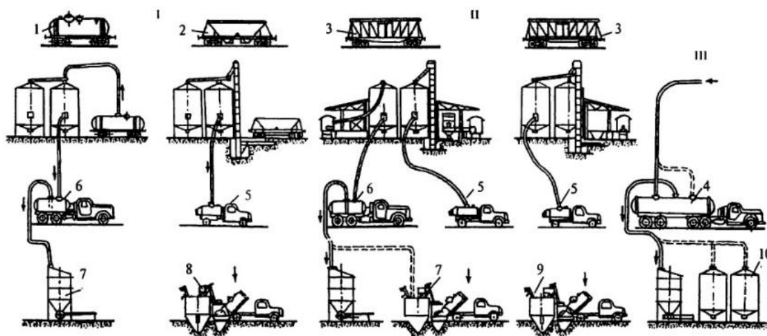
Рис. 6.7. Технологические схемы комплексной механизации выгрузки, погрузки и перевозки цемента на прирельсовых складах емкостью более 300 т и приобъектных складах емкостью более 25 т:
