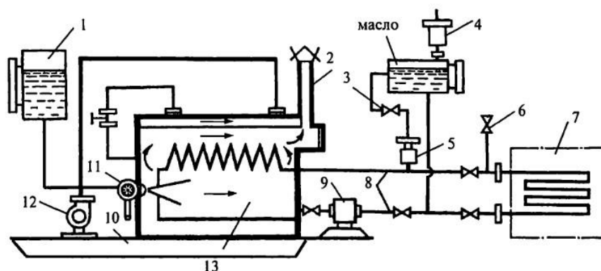
Рис. 4.5. Технологическая схема работы нагревателя цистерны с битумом: 1 – топливный бак; 2 – дымовая труба; 3 – краны регулировки подачи теплоносителя; 4 – силикагельный патрон защиты теплоносителя от влаги; 5 – газосборник; 6 – вентиль подачи сжатого воздуха; 7 – обогреваемые элементы битумного оборудования; 8 – трубопроводы; 9 – насос для перекачки теплоносителя; 10 – опорная рама; 11 – автомобильная форсунка; 12 – вентилятор; 13 – камера нагрева теплоносителя (масла).
