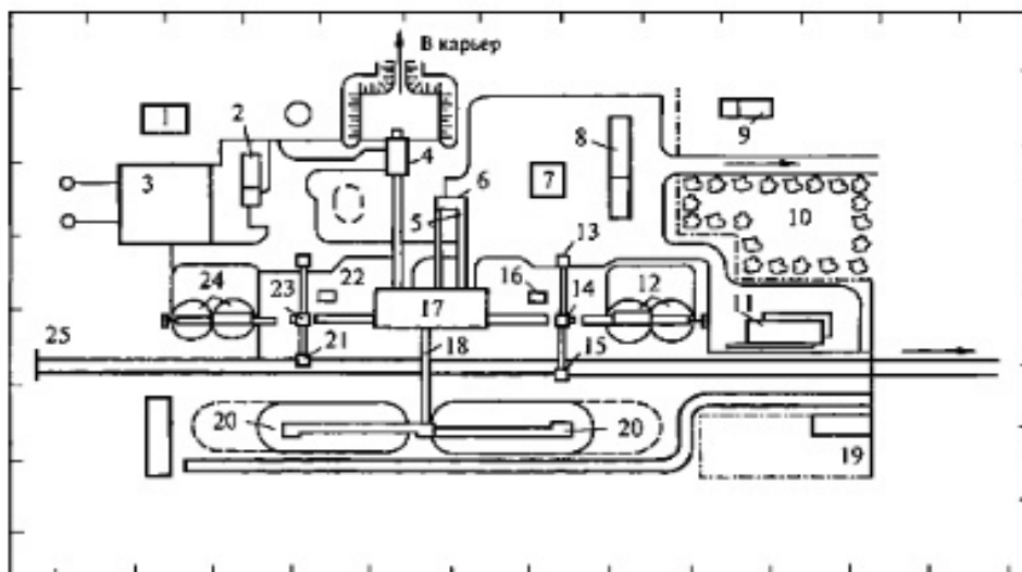
Рис 3.10. Генеральный план гравийно-песчаного КДЗ с раздельной выдачей гравия и песка:
