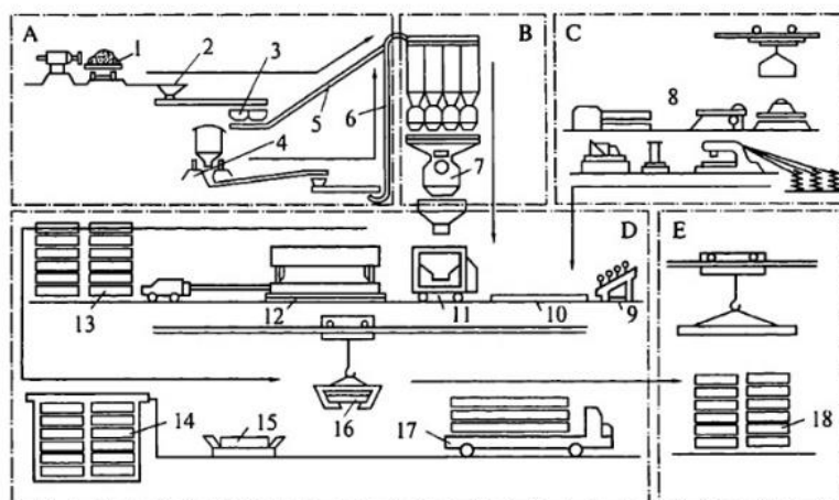
Рис. 6.24. Технологическая схема изготовления железобетонных изделий поточно-агрегатным способом:
