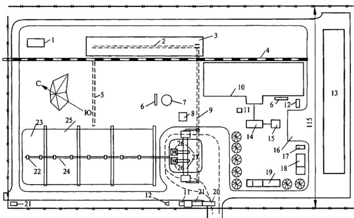
Рис. 5.2. Генеральный план асфальтобетонного завода с двумя смесителями:
