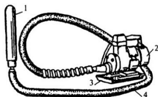
Рис. 6.29. Глубинный вибратор: 1 — виброулава; 2 — электродвигатель; 3 — салазки; 4 — гибкий вал.
