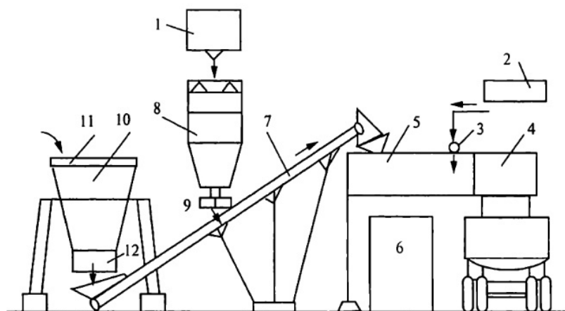
Рис. 5.24. Технологическая схема приготовления укрепленного грунта цементом:
