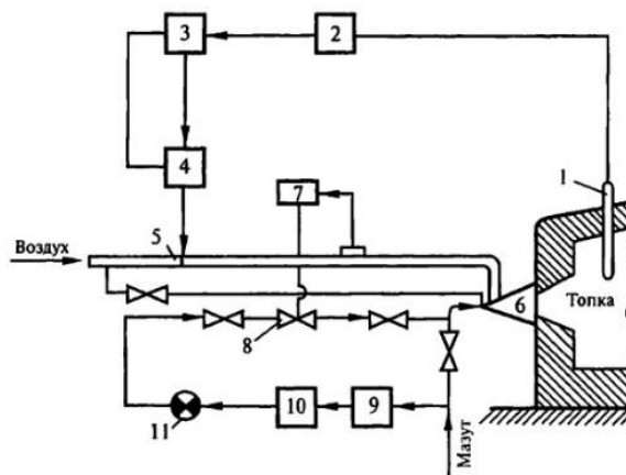
Рис. 7.4. Структурная схема автоматического регулирования теплового режима топки сушильного барабана при подаче жидкого топлива:
