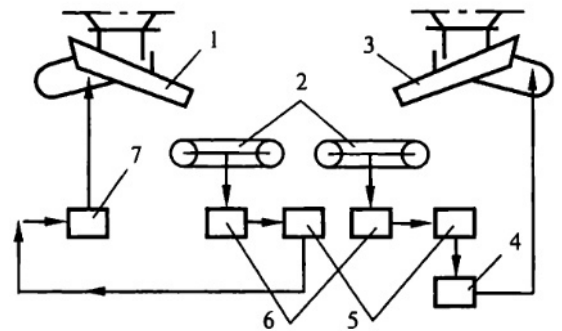
Рис. 7.11. Схема дозирующей установки для обеспечения требуемого соотношения двух компонентов:
