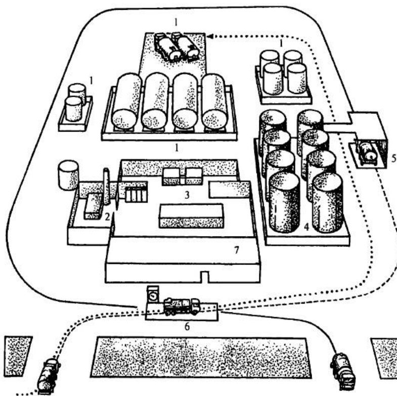
Рис. 4.9. Принципиальная схема эмульсионной базы:
