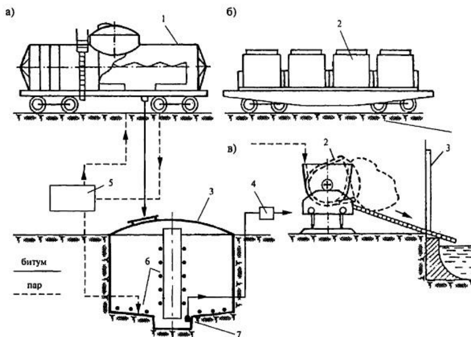
Рис 4.1. Транспортные средства для перевозки битума по железной дороге и разгрузка его на битумной базе:
