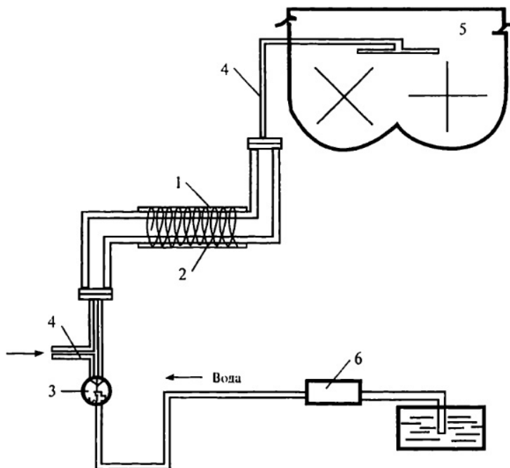
Рис. 5.15а. Схема электромагнитной активации битума: 1 — электромагнитная катушка; 2 — диамагнитная труба; 3 — форсунка; 4 — битумопровод; 5 — смеситель; 6 — водяной насос.
