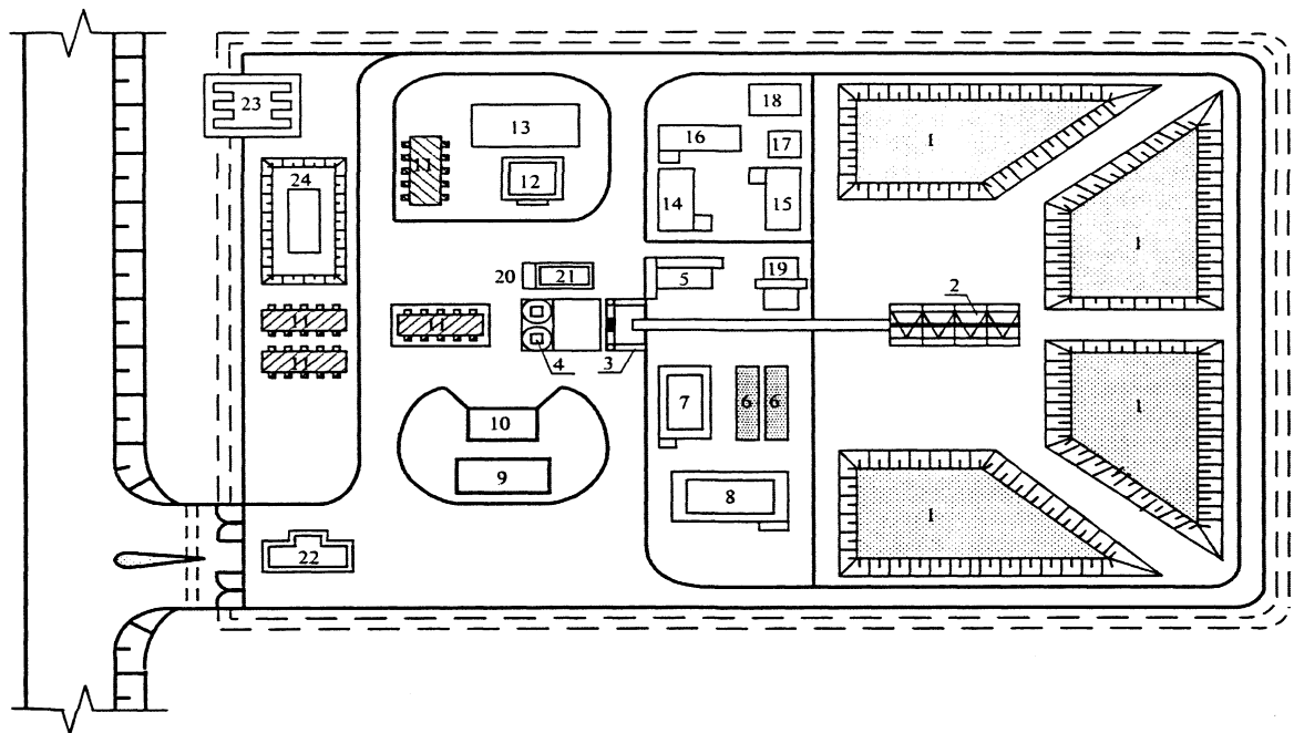
Рис. 3.2. Генеральный план притрассового АБЗ:
