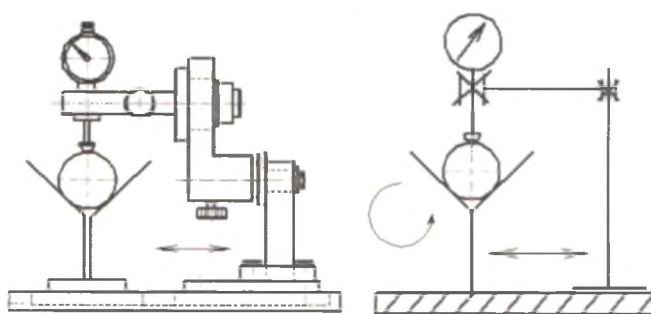
Рисунок 1 – Примеры выполнения схем измерения
