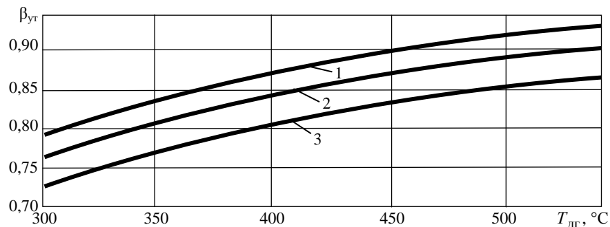
Рис. 3. Зависимость степени утилизации дымовых газов ГТУ от температуры:
