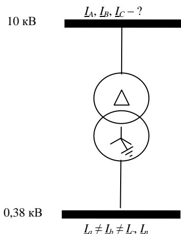
Рис. 2. Трехфазный двухобмоточный трансформатор 10/0,38 кВ
