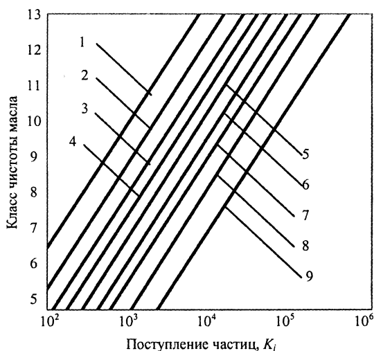
Рис. 1. Зависимость класса чистоты масла от поступления твердых частиц K_i размером 10...25 мкм для разных значений коэффициента отфильтровывания \phi : 1 – \phi = 0,1 ; 2 – 0,2 ; 3 – 0,3 ; 4 – 0,4 ; 5 – 0,5 ; 6 – 0,6 ; 7 – 0,7 ; 8 – 0,8 ; 9 – 0,9
