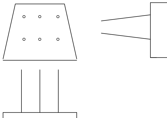
Рис. 5.2. Горизонтальный клиновой вруб
