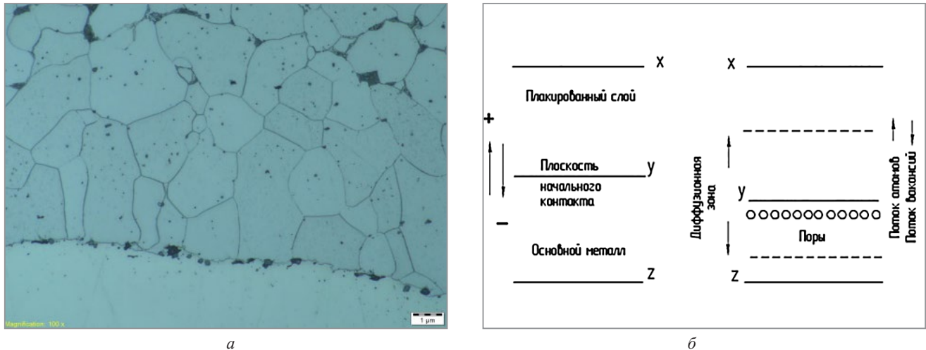
Рис. 3. Диффузионные микropopы в микроструктуре проката (а). \times 100 ; схематическое изображение эффекта Киркендалла (б)
