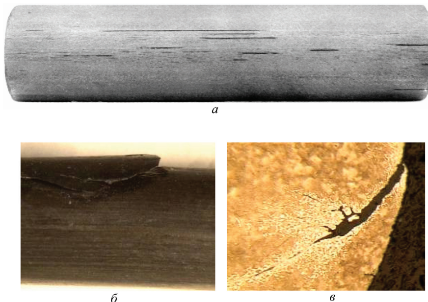
Рис. 1. Раскатанный пузырь: a – внешний вид дефекта на поверхности катанки; б – внешний вид дефекта на поверхности холоднотянутой проволоки; в – микроструктура проволоки в зоне дефекта
