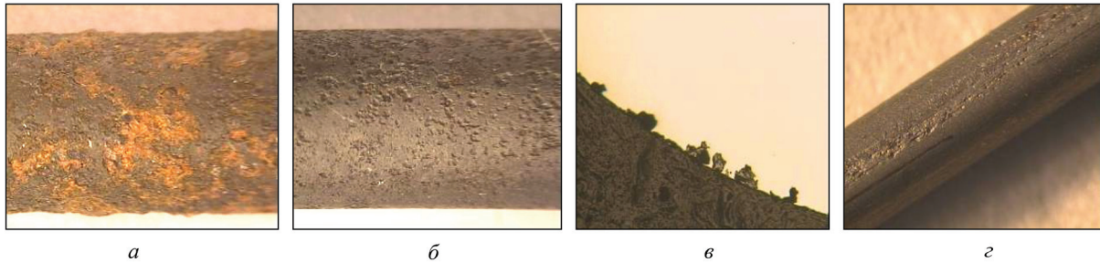
Рис. 7. Коррозия: а – внешний вид дефекта на поверхности катанки; б – внешний вид дефекта на поверхности катанки после травления на участке грубосреднего волочения и травления; в – «разъеденная» поверхность в поперечном сечении микрошлифа; г – внешний вид дефекта на поверхности холоднотянутой проволоки
