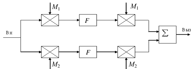
Рис. 1. M_1 = M_0 \sin \omega_M t ; M_2 = M_0 \cos \omega_M t ; F – фильтр НЧ
