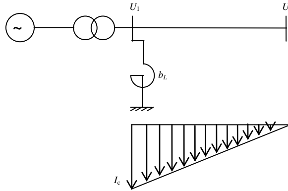
Рис. 1. Распределение емкостных токов вдоль линии U_1 = U_2 = U
