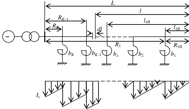
Рис. 2. Распределение емкостных токов вдоль линии с шунтирующими реакторами U_1 = \dots U_K \dots = U_2 = U
