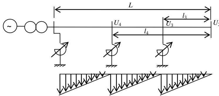
Рис. 3. Распределение емкостных токов вдоль линии с управляющими шунтирующими реакторами U_1 = U_4 = U_3 = U_1
