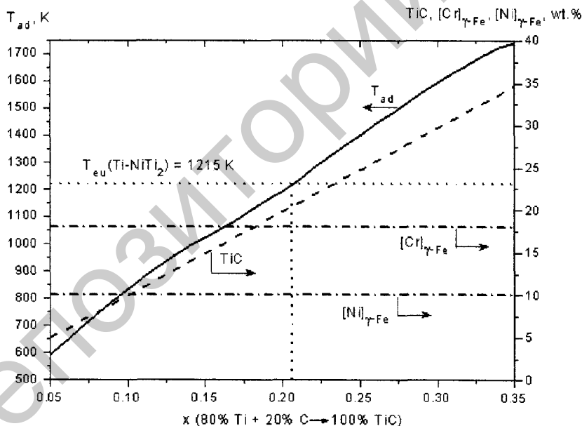
Рис. 4. Результаты термодинамического моделирования экзотермического взаимодействия в составе 4 на основе Fe: адиабатическая температура, доля упрочняющей фазы ( TiC ) и содержание хрома и никеля в \gamma -твердом растворе на основе железа
