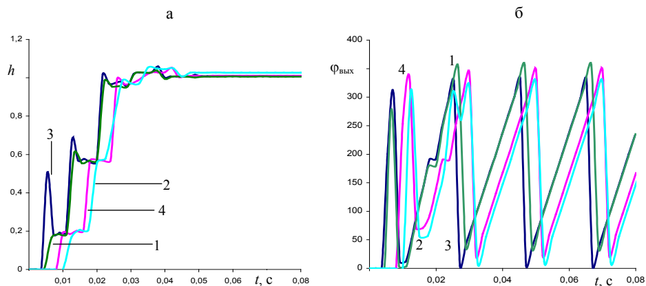
Рис. 5. Реакция ФОС на синусоидальный входной сигнал: а – изменение амплитуды; б – фазы выходного сигнала; 1 – n = 10 ; \Delta t = 0,00222 с; f_{cp} = 120 Гц; 2 – 10; 0,0025 с; 120 Гц; 3 – 12; 0,00181 с; 125 Гц; 4 – 12; 0,002 с; 125 Гц
