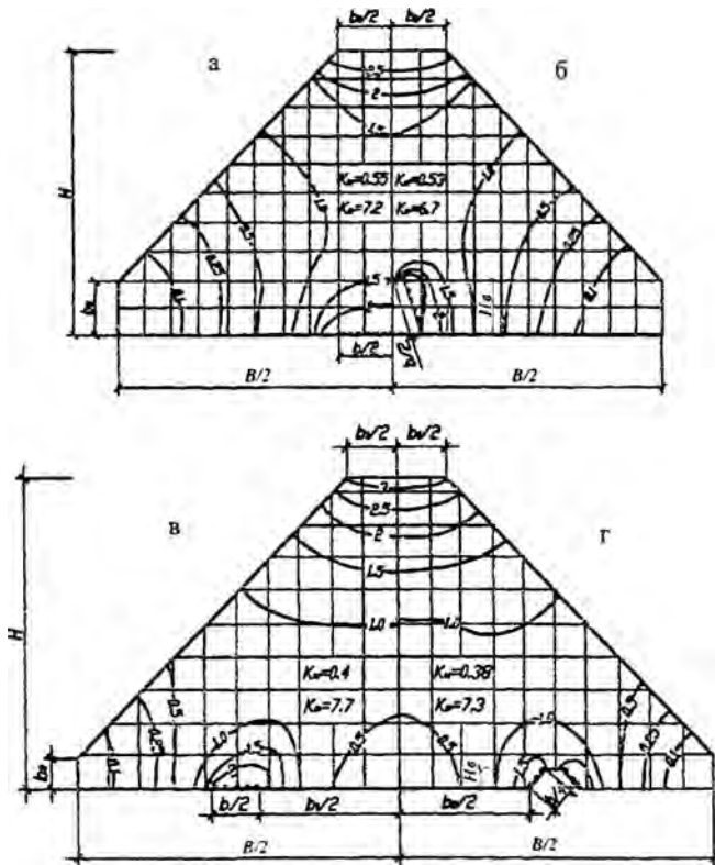
Рис. 2. Поле относительных скоростей w_i/w_{cp} в поперечном сечении некоторых типов буртов
