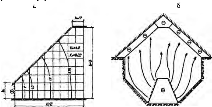
Рис. 3. а – поле скоростей w_i/w_{cp} фильтрации воздуха при расположении приточного и вытяжного воздуховодов в основании; б – схема бурта по [4]
