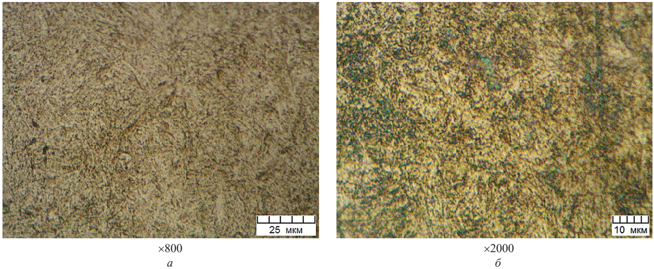
Рис. 2. Микроструктура стали 30MnB4: a – структура после закалки; б – структура после отпуска
