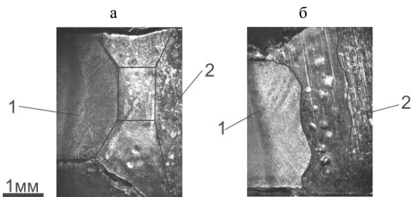
Рис. 2. Макроструктура сварного шва при различных энерговыкладах: а – удельная энергия 681,8 Дж/мм 2 ; б – 833,3 Дж/мм 2 ; 1 – основание; 2 – сегмент
