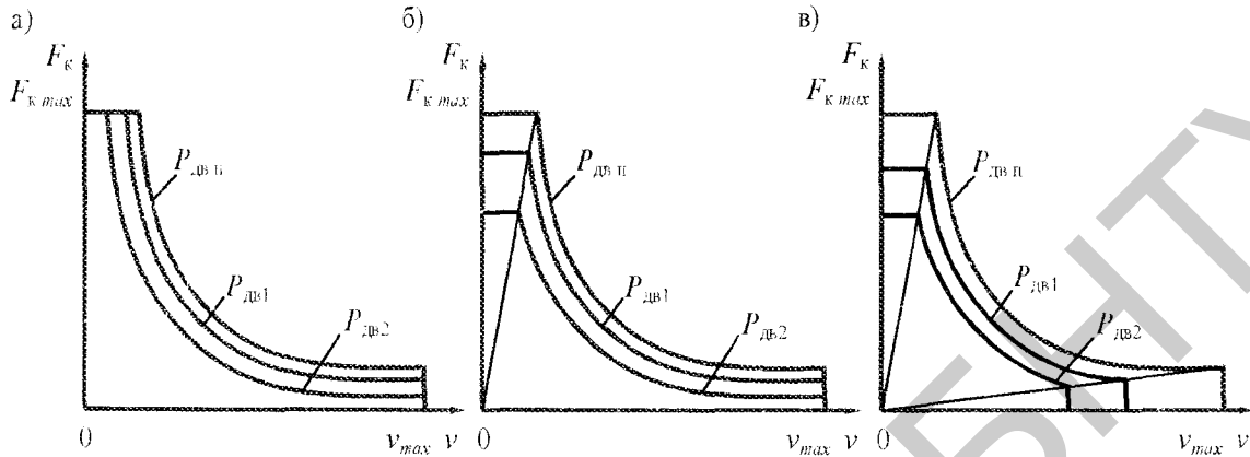
Рис. 2. Семейство тяговых характеристик подвижного состава: P_{дв.п} , P_{дв.1} , P_{дв.2} — значения мощности двигателя, соответствующие предельной и частичным характеристикам
