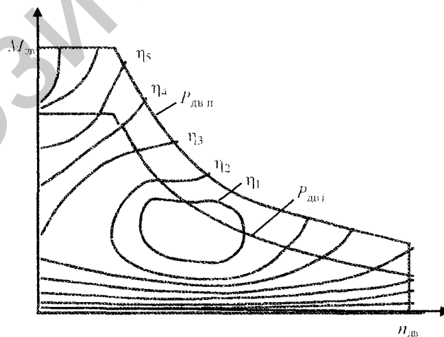
Рис. 3. Тяговые характеристики электродвигателя при постоянных значениях P_{\text{дв } n} , P_{\text{дв } i} мощности и постоянных значениях \eta_i ( \eta_i > \eta_{i+1} ) коэффициента полезного действия
