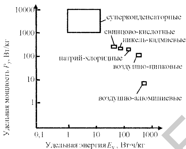
Рис. 4. Удельные параметры АЭУ
