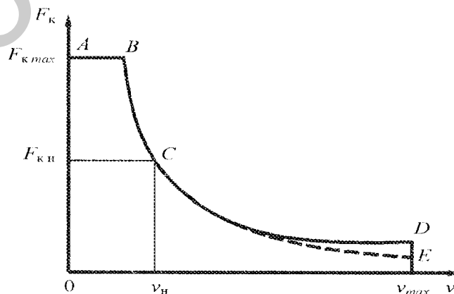
Рис. 1. Предельная тяговая характеристика подвижного состава с электрической трансмиссией
