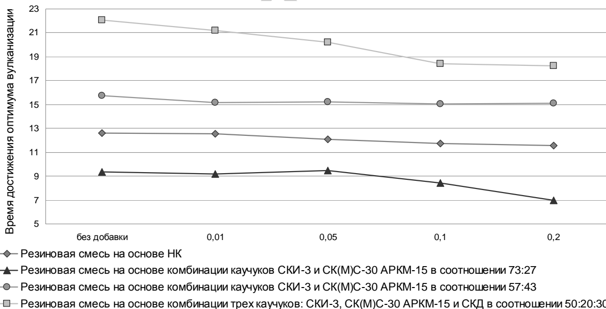
Рисунок 1 – Время достижения оптимума вулканизации для смесей на основе каучуков общего назначения с различными дозировками модифицирующей добавки
