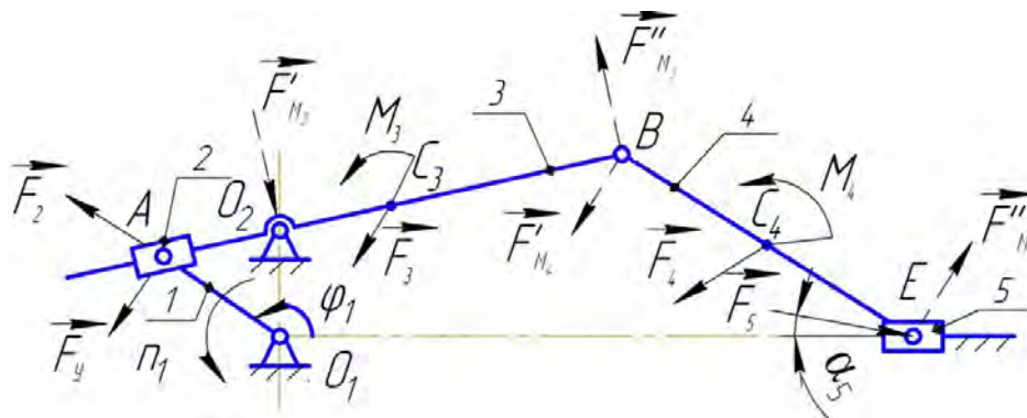
Рысунк.2 - Кінематычная схема механізма і сілавыя фактары
