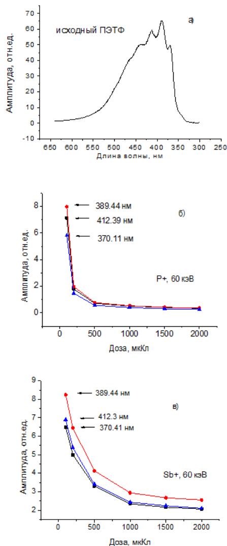
Рисунок 1 – Зависимость амплитуды спектра люминесценции с узкими линиями (а) в образцах ПЭТФ от дозы облучения ионами фосфора (б) и сурьмы (в)
