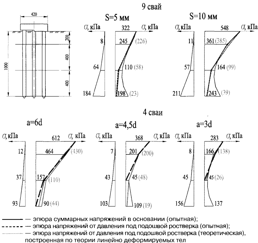
Рис. 4. Экспериментальные и теоретические эпюры распределения напряжений в основании ростверка
