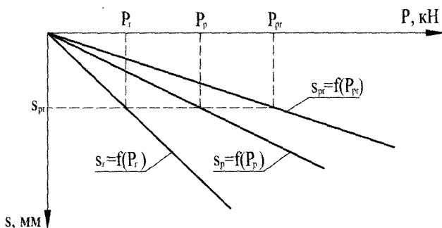
Рис. 7. Графический способ определения осадки свайного фундамента с несущим ростверком
