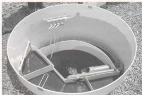
Рис. 5. Установка для очистки сточных вод заводского изготовления
