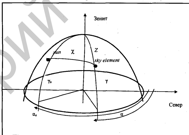
Рис. 2. Углы, определяющие положение солнца и элемента неба
