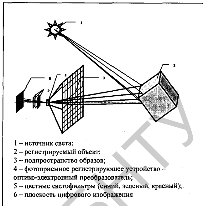
Рис. 1. Принцип формирования цифрового изображения трехмерного объекта
