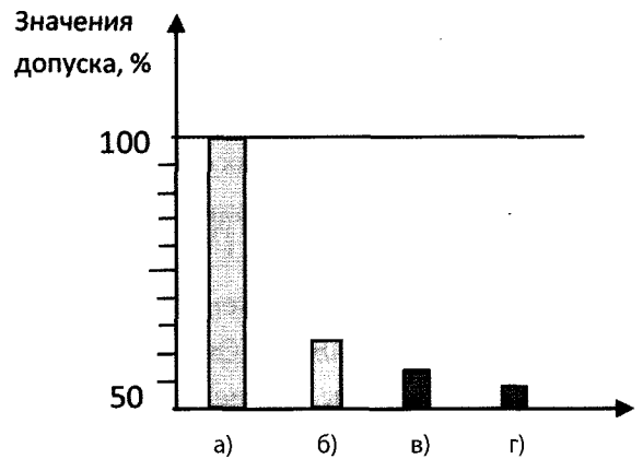
Рисунок 4 – Значения допусков формы по отношению к допуску размера (класс точности «грубый») при разных видах нормирования общих допусков формы и расположения поверхностей:
