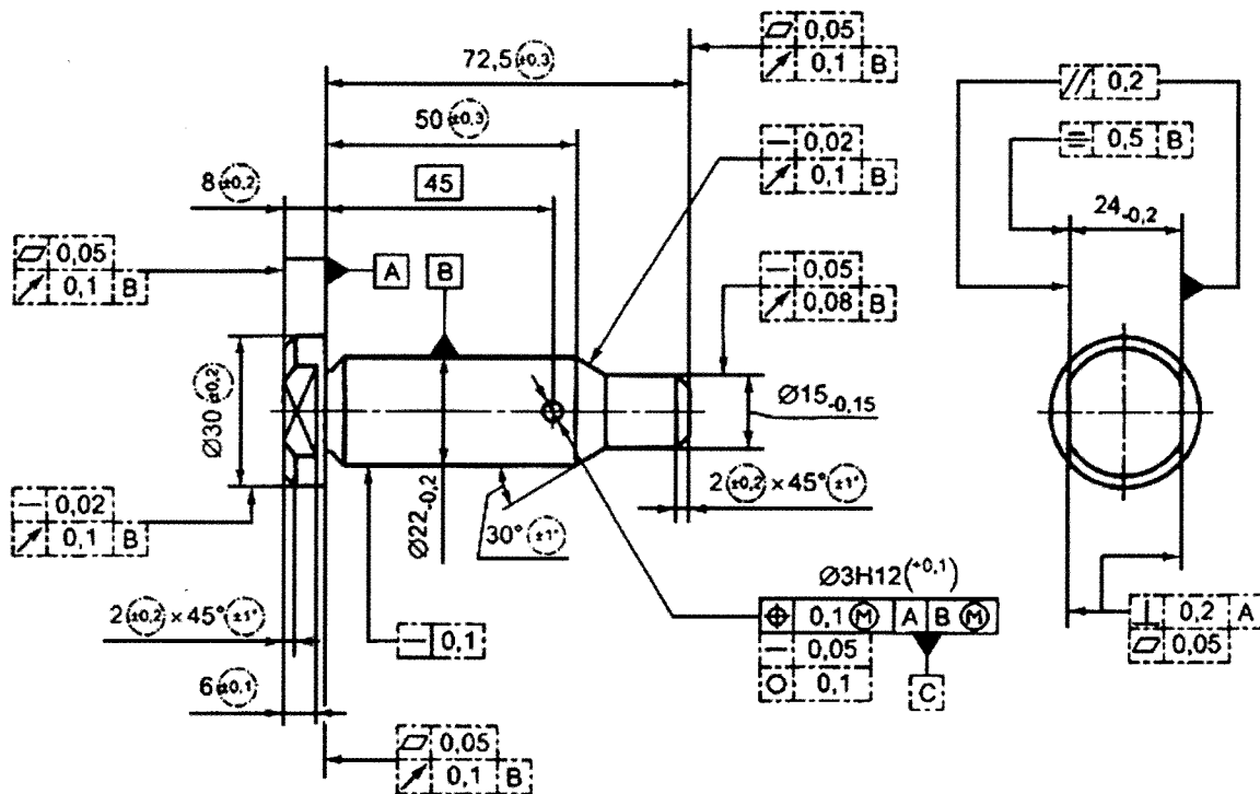
Рисунок В.2 Интерпретация общих допусков
