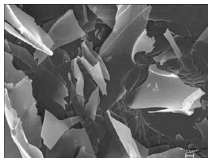
Рис. 4. Фрагмент структуры вспученной щелочно-силикатной сырьевой смеси, содержащей 5 % буры
