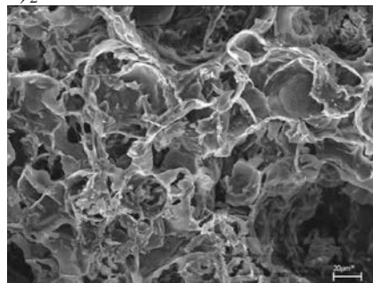
Рис. 3. Фрагмент структуры вспученного образца, полученного из жидкого стекла, содержащего 5 % Al_2(SO_4)_3
