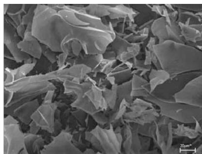
Рис. 1. Фрагмент структуры вспученного образца, полученного из жидкого стекла
