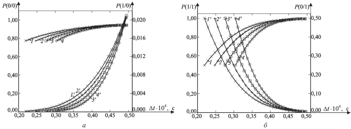
Рис. 2. Зависимости переходных вероятностей P(0/0) , а, 1–4, P(1/0) , а, 1'–4', P(1/1) , б, 1–4, P(0/1) , б, 1'–4', от времени однофотонной передачи: N_1 = 1 , N_2 = 7 , n_t = 10^3 \text{ с}^{-1} , \tau_b = 100 \text{ мкс} ; средняя длительность мертвого времени: 1 и 1' – \tau_d = 0 ; 2 и 2' – \tau_d = 5 \text{ мкс} ; 3 и 3' – \tau_d = 10 \text{ мкс} ; 4 и 4' – \tau_d = 15 \text{ мкс}
