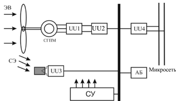
Рис. 3. Схема интегрированной установки на основе солнечных батарей:
