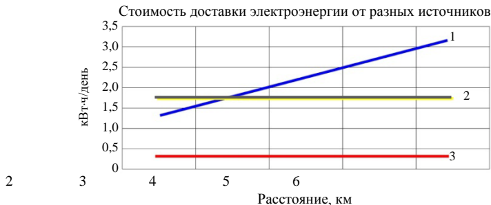
Рис. 5. Стоимость киловатт-часа в зависимости от расстояния: 1 – сеть электропитания; 2 – дизель-генераторы; 3 – солнечная энергия
