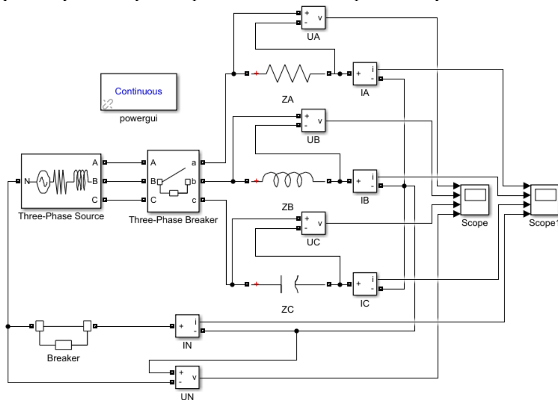
Рисунок 1. Модель исследуемой трехфазной электрической цепи
