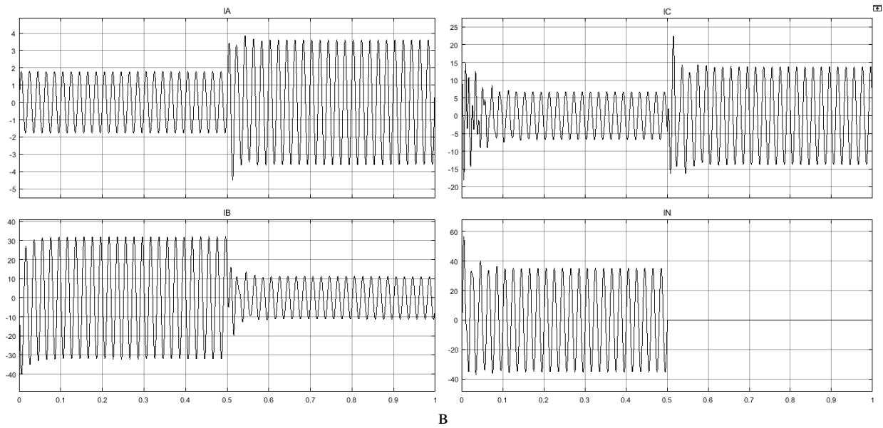
Рисунок 4. Осциллограммы токов при протекании переходного процесса
