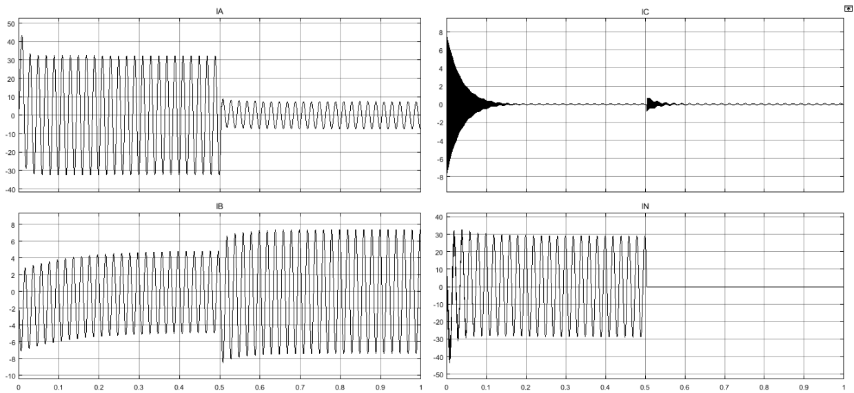
Рисунок 2. Осциллограммы токов при протекании переходного процесса
