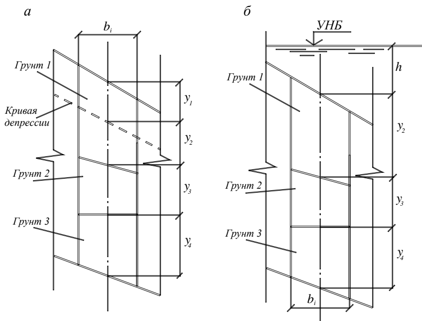
Рис. 4.5. Схема к определению веса отсека: а – при отсутствии воды над отсеком; б – при наличии воды над отсеком
