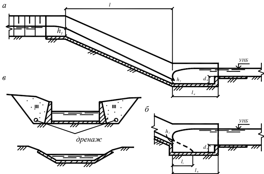
Рис. 5.8. Быстроток: а – без стенки падения; б – со стенкой падения; в – примеры поперечных сечений лотка быстротока
