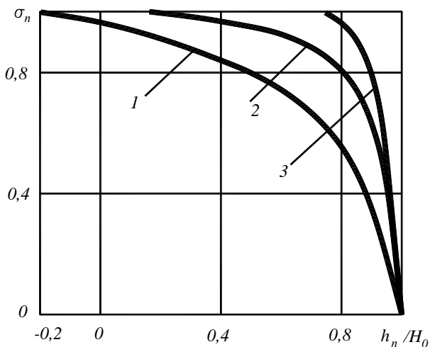
Рис. 5.2. График для определения коэффициента подтопления водослива: 1 – вакуумного; 2 – безвакуумного практического профиля; 3 – с широким порогом
