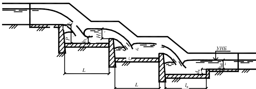
Рис. 5.11. Многоступенчатый перепад
