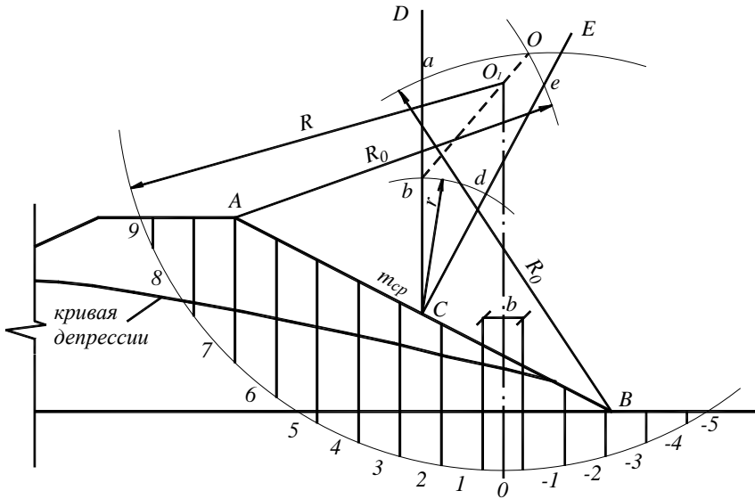
Рис. 4.4. Схема к расчету устойчивости низового откоса
