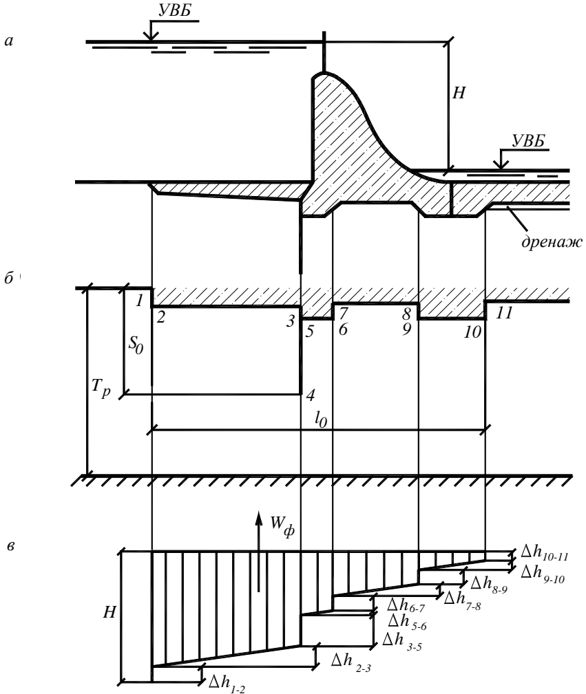
Рис. 5.5. Схема к расчету фильтрации в основании бетонной плотины: а – схема подземного контура; б – расчетная схема подземного контура плотины; в – эпюра фильтрационного давления на подошву плотины
