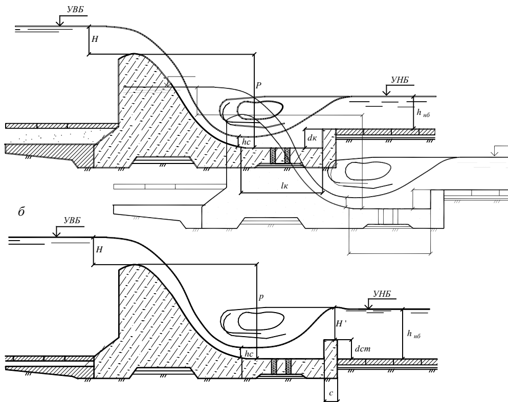
Рис. 5.3. Схемы к расчету донного режима сопряжения бьефов: а – с водобойным колодцем; б – с водобойной стенкой
