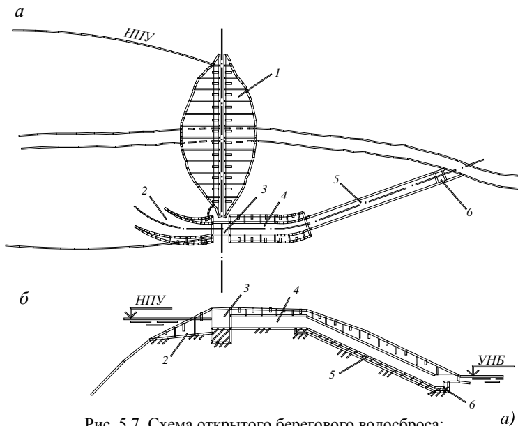
Рис. 5.7. Схема открытого берегового водосброса:
