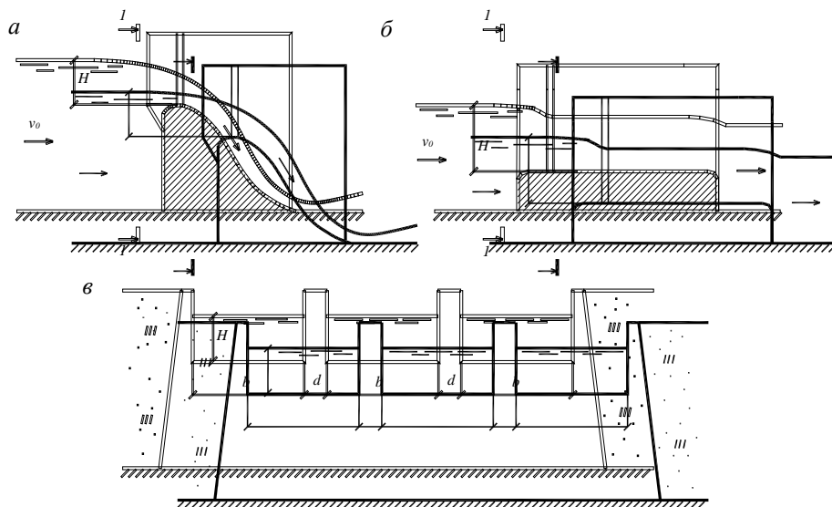
Рис. 5.1. Гидравлический расчет водосливной плотины: a – водослив практического профиля; б – водослив с широким порогом; в – вид 1 – 1
