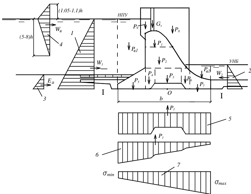
Рис. 5.6. Статические расчеты бетонной плотины:
