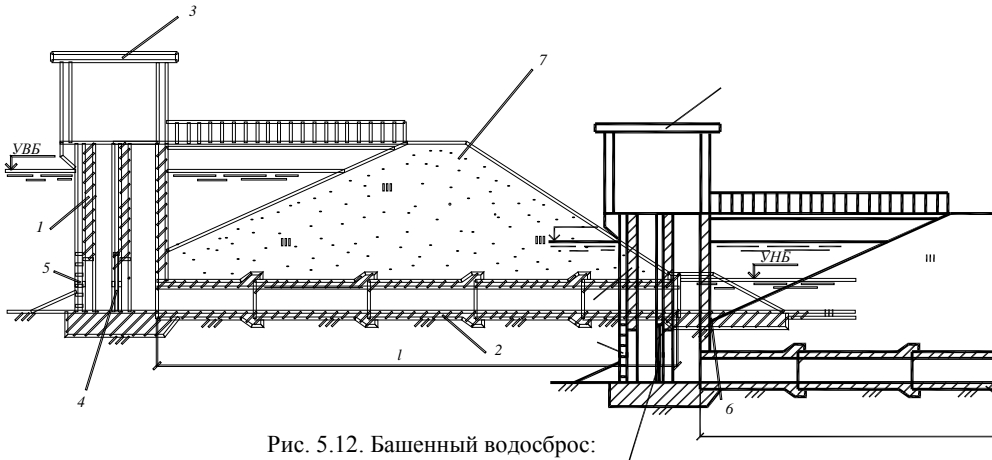
Рис. 5.12. Башенный водосброс:
