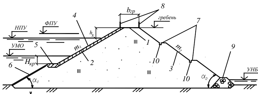
Рис. 4.1. Поперечный профиль грунтовой плотины:
