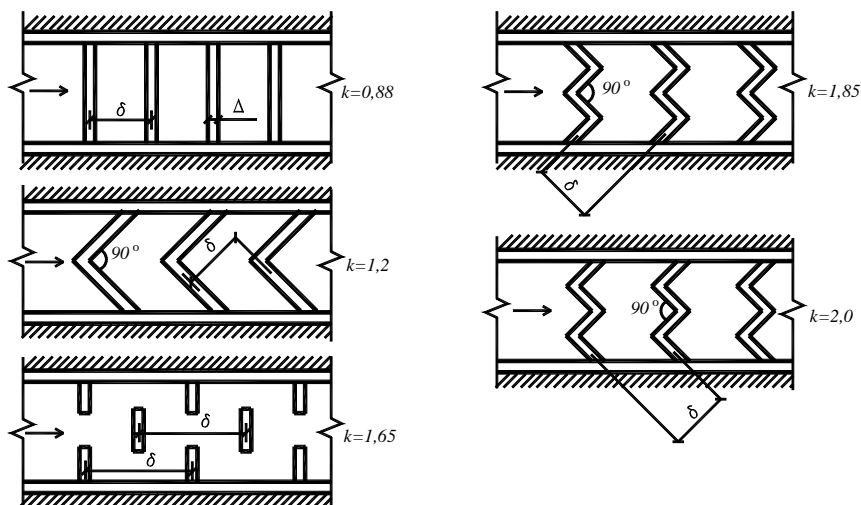
Рис. 5.9. Типы усиленной шероховатости на быстротоке
