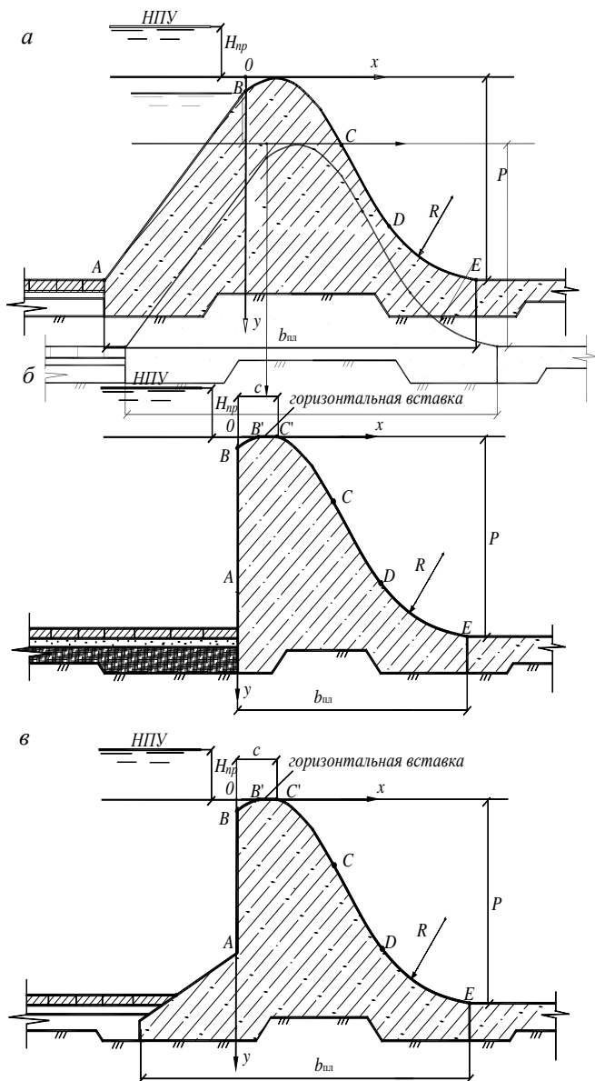
Рис. 5.4. Построение профиля безвакуумного водослива практического профиля: a – без горизонтальной вставки на гребне; б, в – с горизонтальной вставкой на гребне
