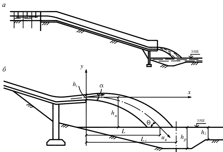
Рис. 5.10. Консольный перепад: а – общий вид; б – схема к расчету дальности отброса струи
