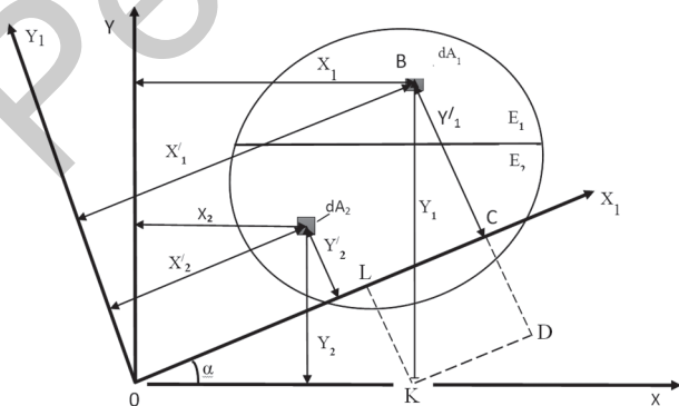
Рисунок — Осевое сечение, состоящее из двух различных материалов
