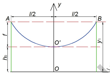
Рис. 1. Кривая провисания провода: l – длина пролета; f – стрела провеса; h_0 – габарит (расстояние от нижней точки провода до оси x ); y_1 – высота опоры Fig. 1. The curve of wire sag: l – length of span; f – sag; h_0 – dimension (distance from the lowest point of the wire to the x -axis); y_1 – height of the pillar
