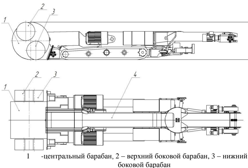
Рис. 1 – Комбайн для отработки краевых зон
