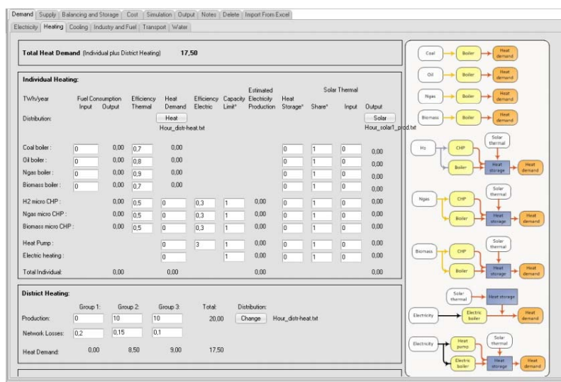
Рисунок 3 – Страница модели EnergyPLAN по введению данных по теплотреблению по видам потребителей
