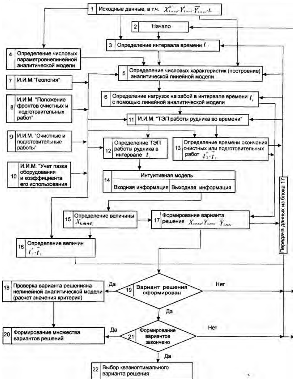
Рис. 2. Блок-схема алгоритма управления производственной деятельностью калийных рудников с помощью интуитивных математических моделей
