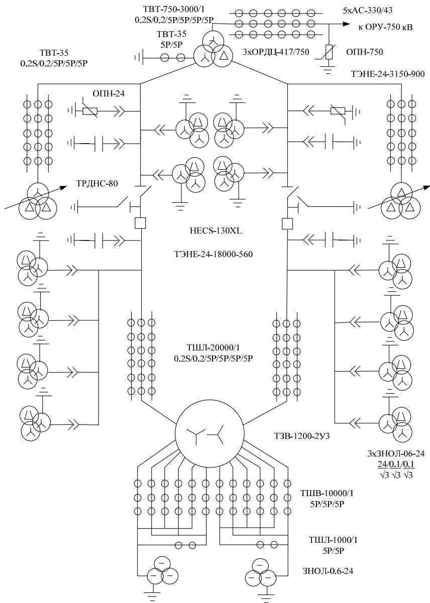
Рис. 8.3. Результаты выбора токоведущих частей и электрических аппаратов цепей генератора 1200 МВт
