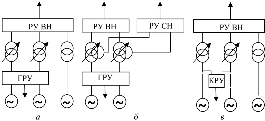
Рис. 5.1. Структурные схемы ТЭЦ
