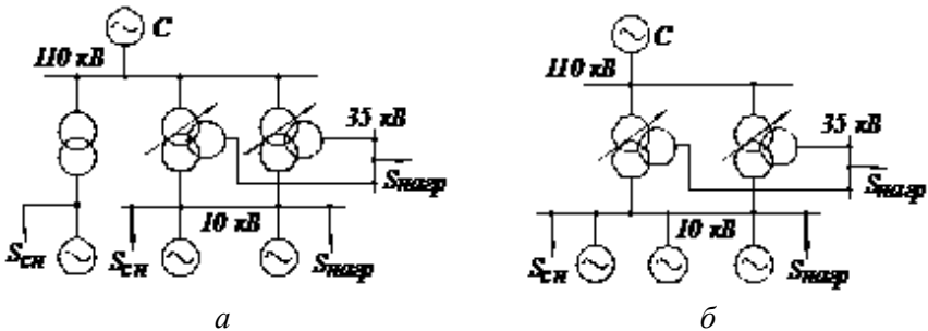
Рис. 5.2. Схемы выдачи мощности ТЭЦ к примеру 6: а – первый вариант; б – второй вариант
