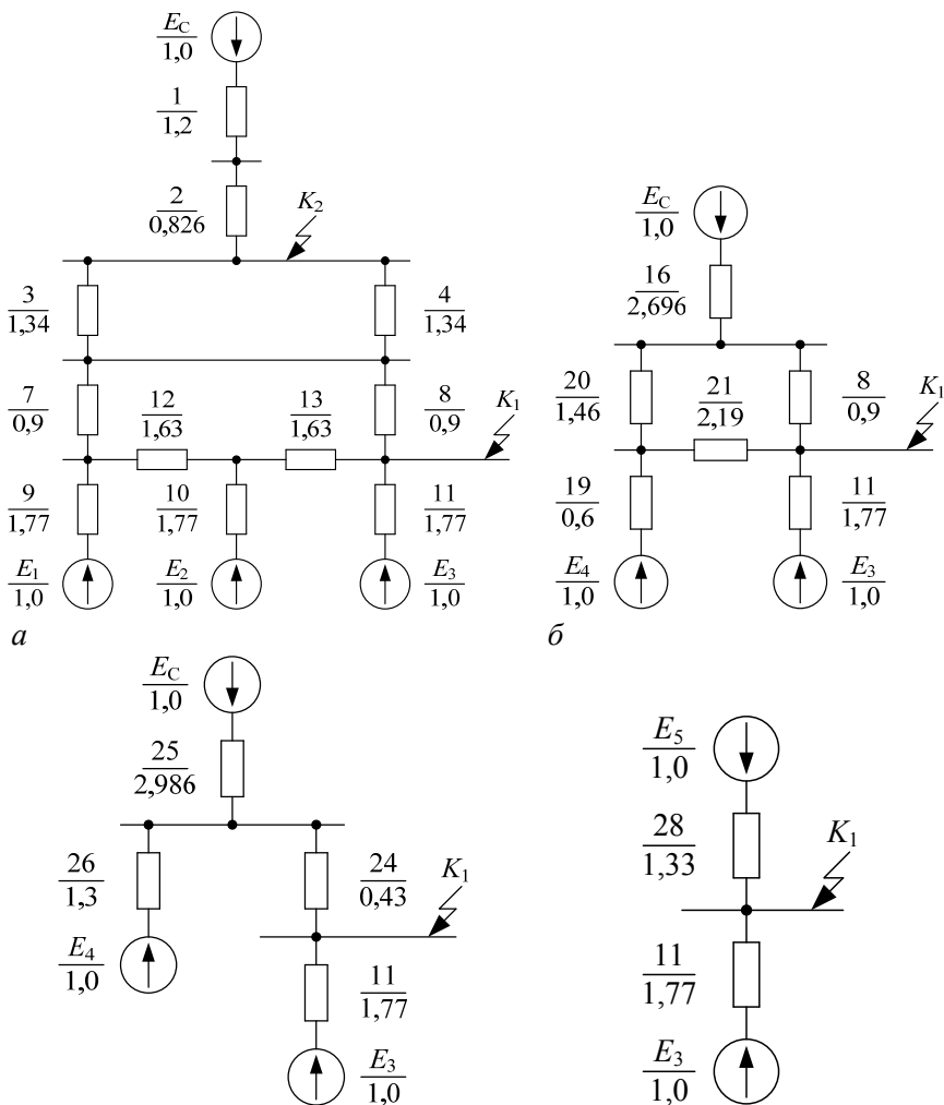
Рис. 6.2. Эквивалентная схема замещения и пути ее преобразования
