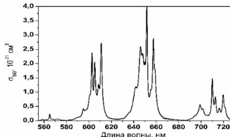
Рисунок 2 – Спектр вынужденного излучения кристалла \text{Sm}^{3+}:\text{KYW} (поляризация E||N_m )
