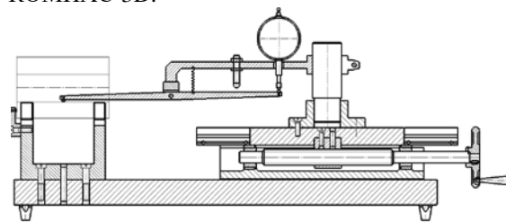
Рисунок 1 - Контрольное приспособление для контроля полного радиального биения отверстия
