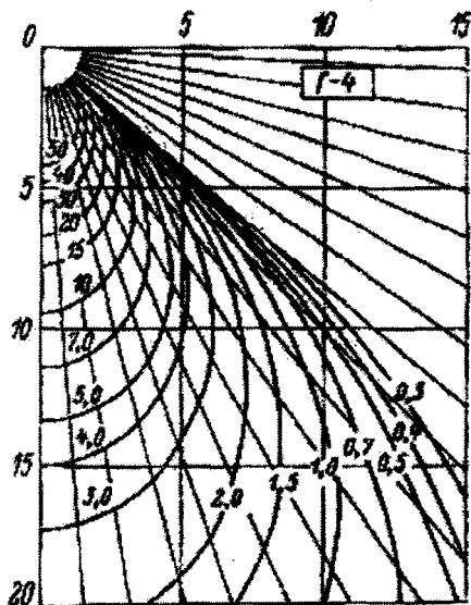
Рис. П6. Пространственные изолюксы условной горизонтальной освещенности от светильников с КСС типа Г-4
