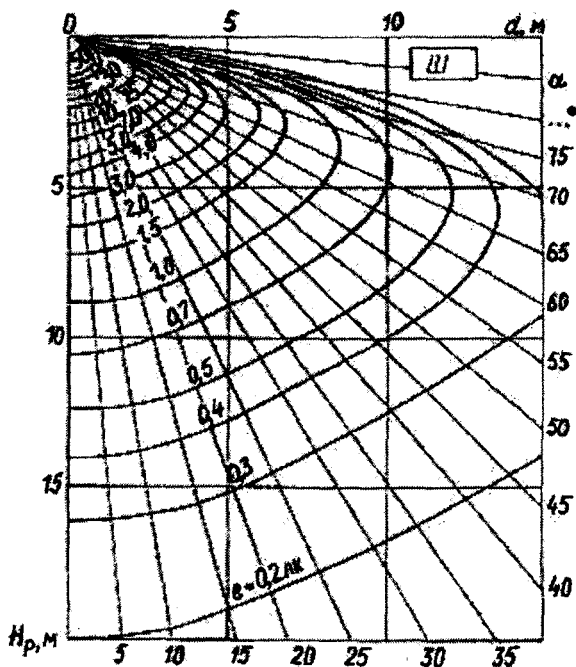
Рис. П17. Пространственные изолюксы условной горизонтальной освещенности от светильников с КСС типа Ш
