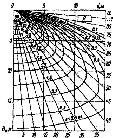
Рис. П14. Пространственные изолюксы условной горизонтальной освещенности от светильников с КСС типа J
