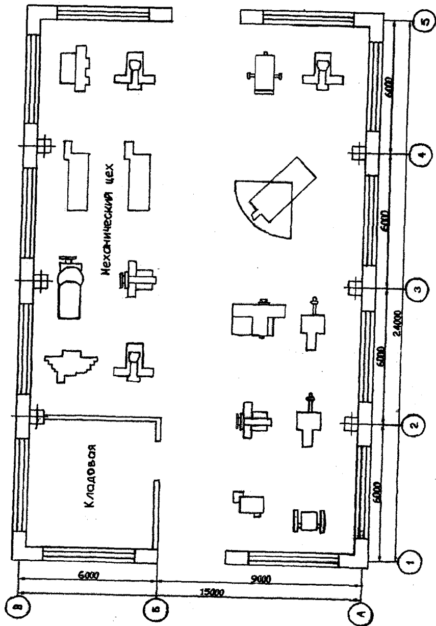
Рис. 5.1. План цеха с расстановкой технологического оборудования
