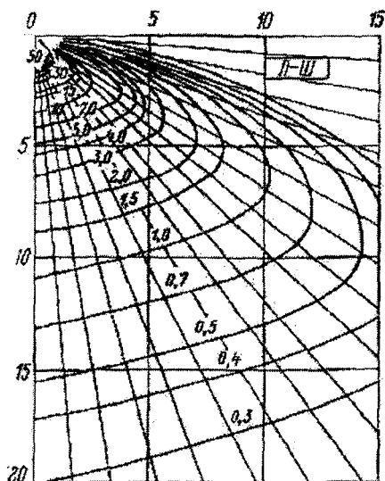
Рис. П15. Пространственные изолюксы условной горизонтальной освещенности от светильников с КСС типа Л-Ш
