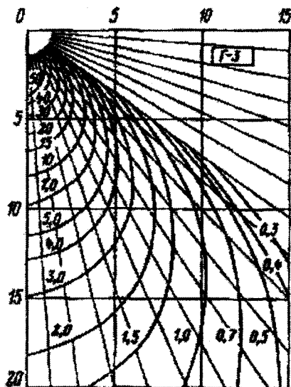
Рис. П5. Пространственные изолюксы условной горизонтальной освещенности от светильников с КСС типа Г-3
