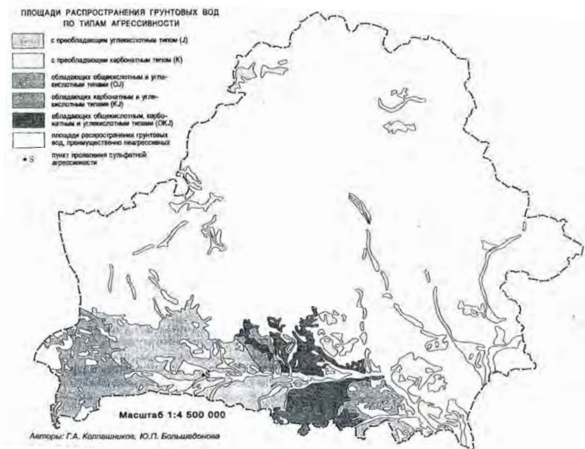
Рис. 3.12. Карта-схема агрессивности грунтовых вод Беларуси
