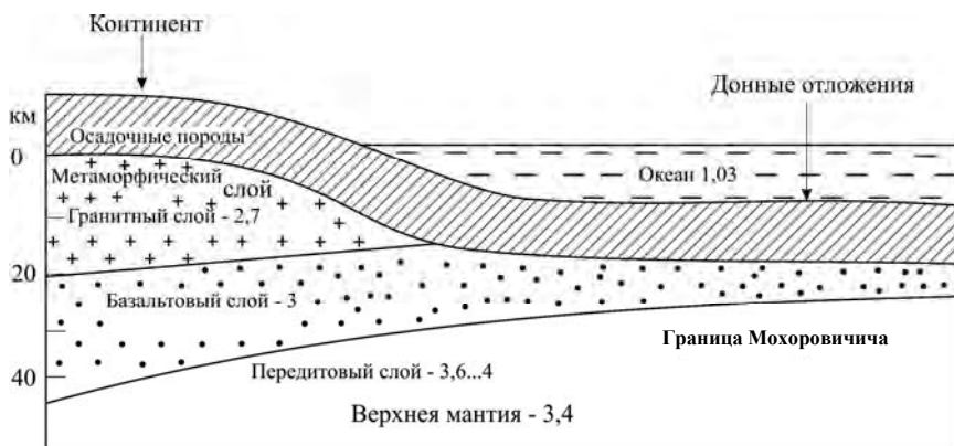
Рис. 1.3. Строение земной коры (с указанием плотностей материалов, т/м 3 )
