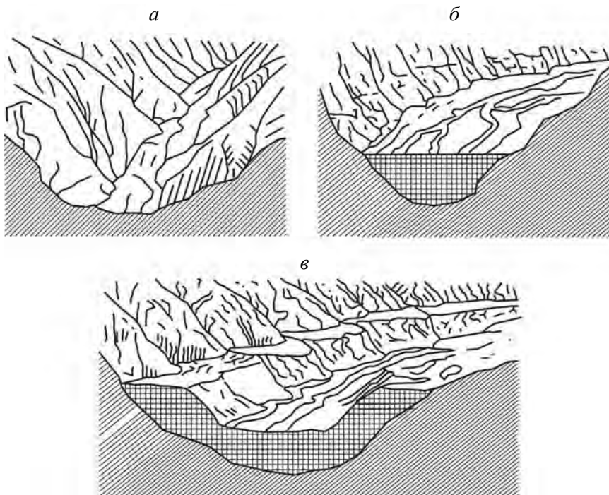
Рис. 1.10. Процесс формирования аккумулятивных террас
