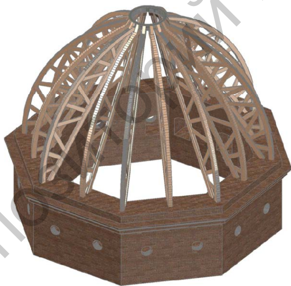
Рисунок 3 – Трехмерная модель купольного покрытия башни
