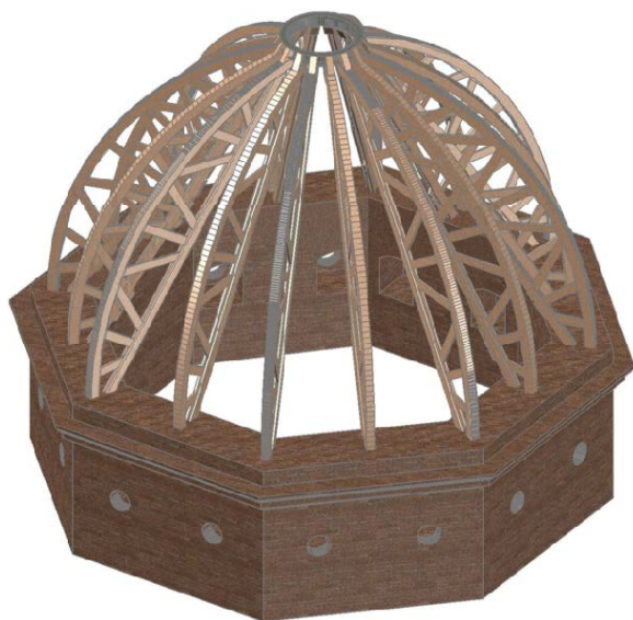
Рисунок 3 – Трехмерная модель купольного покрытия башни
