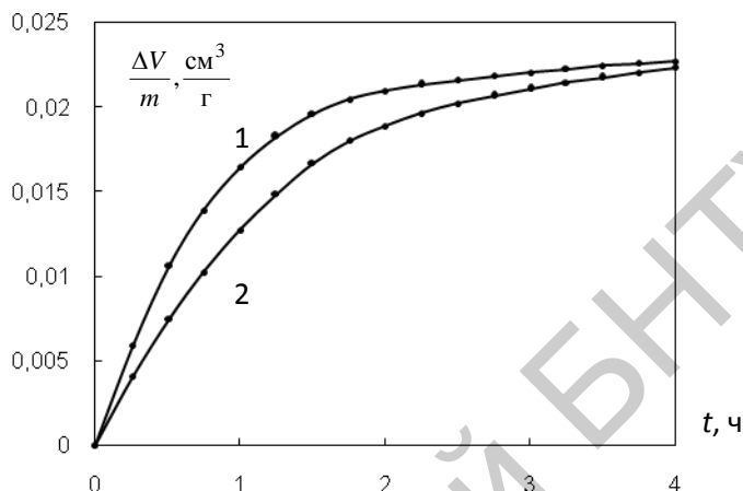
Рис. 1. Зависимости изменения удельного объема \Delta V/m пор от времени содержания в жидкости: 1—10% серной кислоте; 2—дистиллированной воде.
