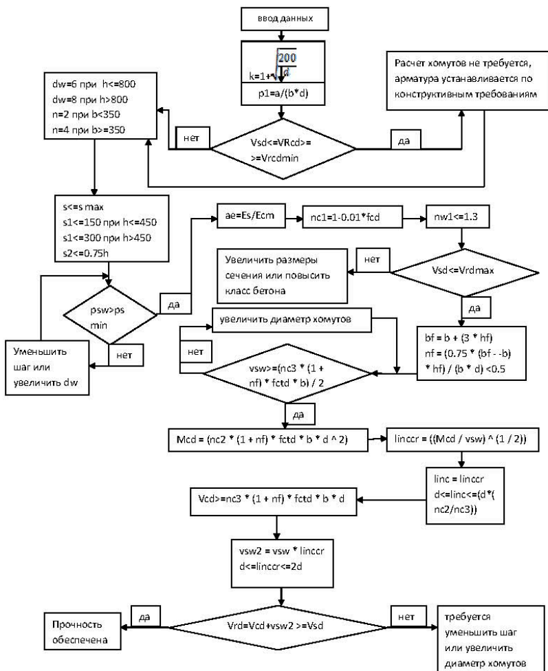
Структура 1. Расчет наклонных сечений.
