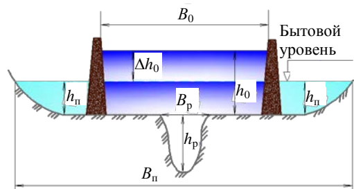
Рис. 1. Схема к расчету обвалования реки Fig. 1. Scheme for calculation of river regulation
