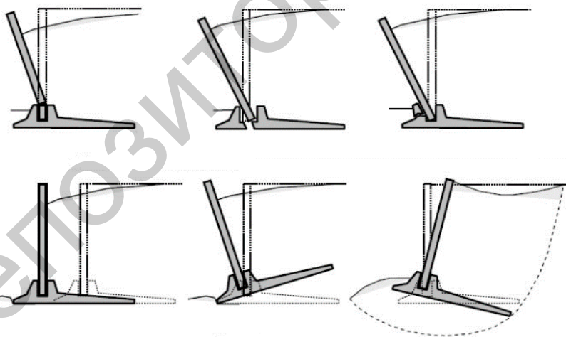
Рисунок 1 – Схемы потери прочности и устойчивости тонких подпорных стен (уголкового профиля)
