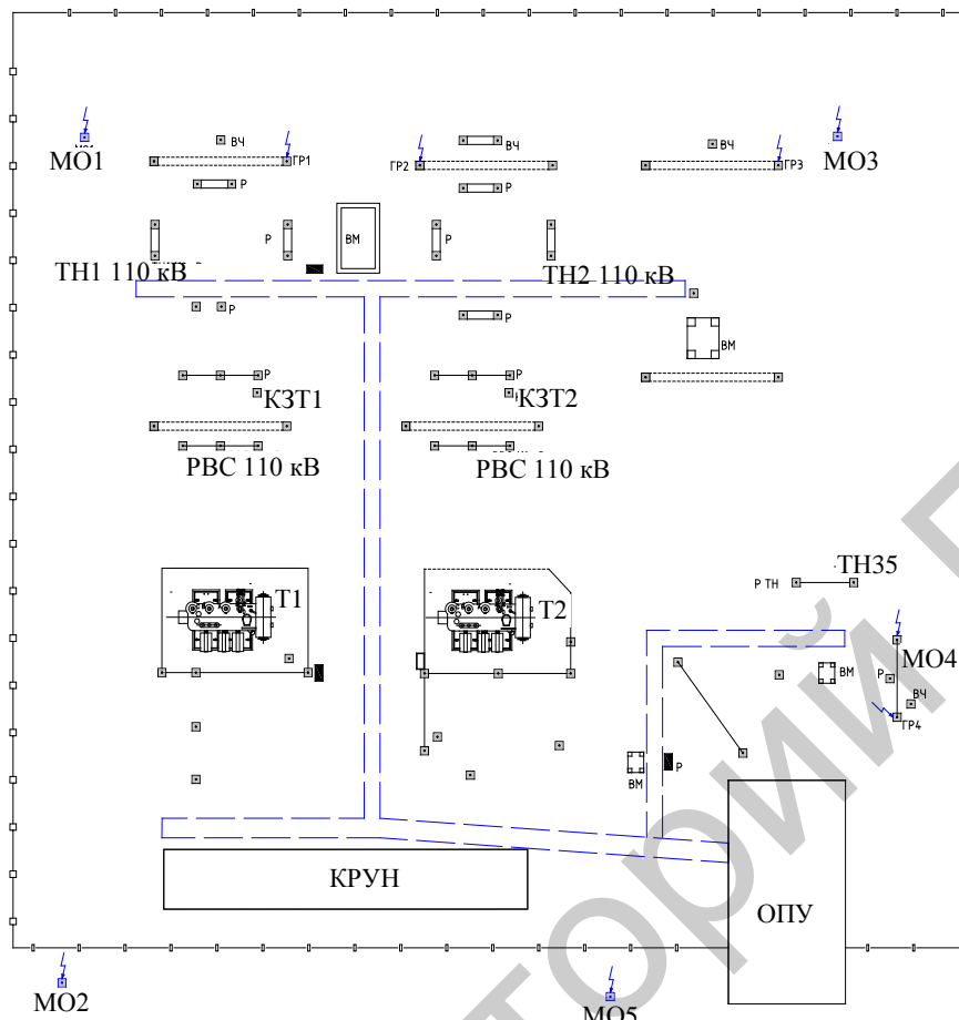
Рис. 2. План подстанции
