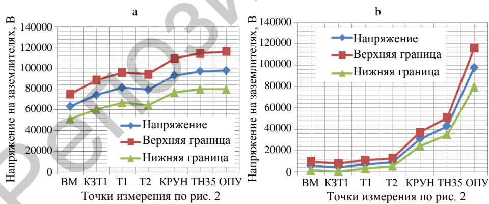
Рис. 3. Результаты измерений и расчетов напряжений на заземляющем устройстве при имитации ударов молнии в молниеотвод MO1 относительно: а – MO1; б – оперативного пункта управления
