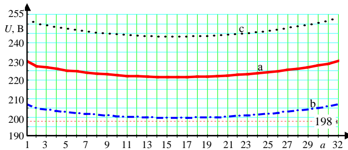
Рис. 5. Графики распределения напряжений в точках осветительной линии для фазы А, построенные для режимов а, б, с при сечении жилы кабеля S = 4 \text{ мм}^2
